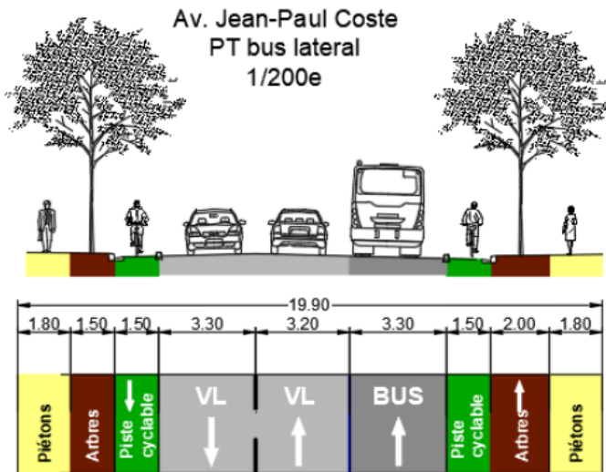
Coupe de principe section 1
