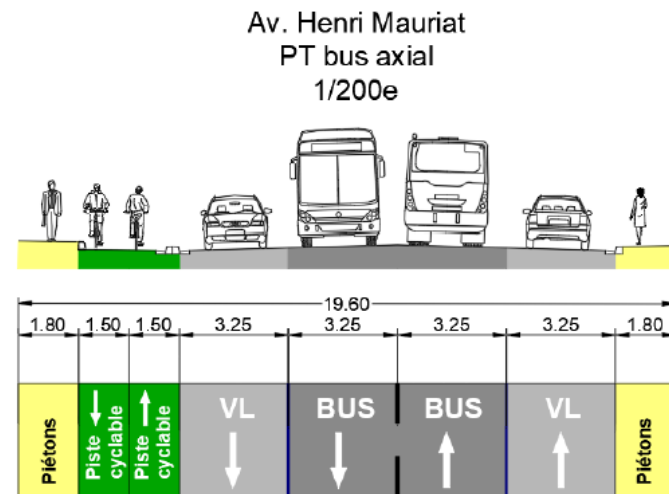
Coupe de principe section 2
