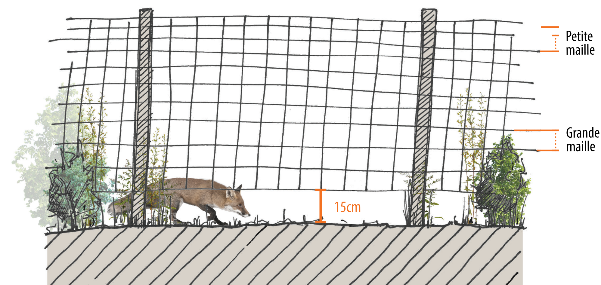
Schéma de la clôture « Ursus » placée à l'envers, 15cm au dessus du sol pour faciliter le passage de la moyenne et petite faune
